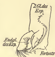
Fig. 4. E. hebes ♂, Distalende des linken 5. B. ( 100\times .)
