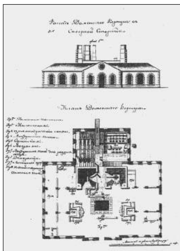
Фасад і план доменного цеху Луганського ливарного заводу 19 ст.
