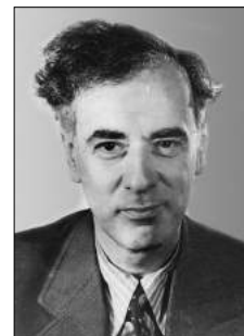
Л.Д. Ландау.
