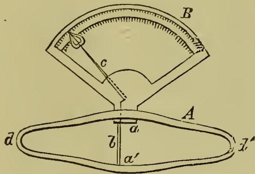
FIG. 24. DYNAMOMETER.
