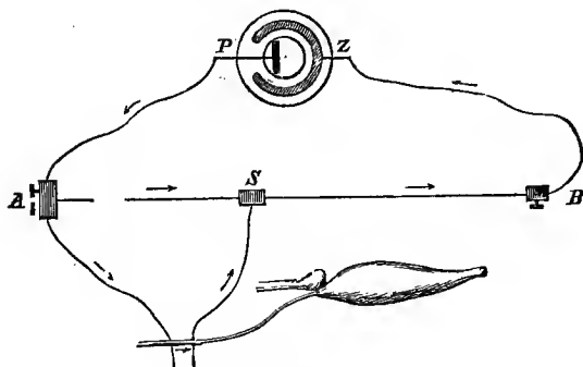
FIG. 35. RUEOCHORD.
