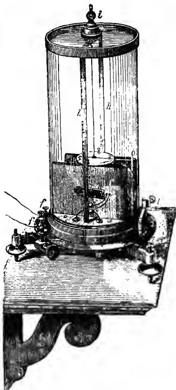
FIG. 37. A MULTIPLIER.
