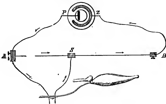
FIG. 32. RHEOCHORD.
