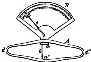
FIG. 24. DYNAMOMETER.
